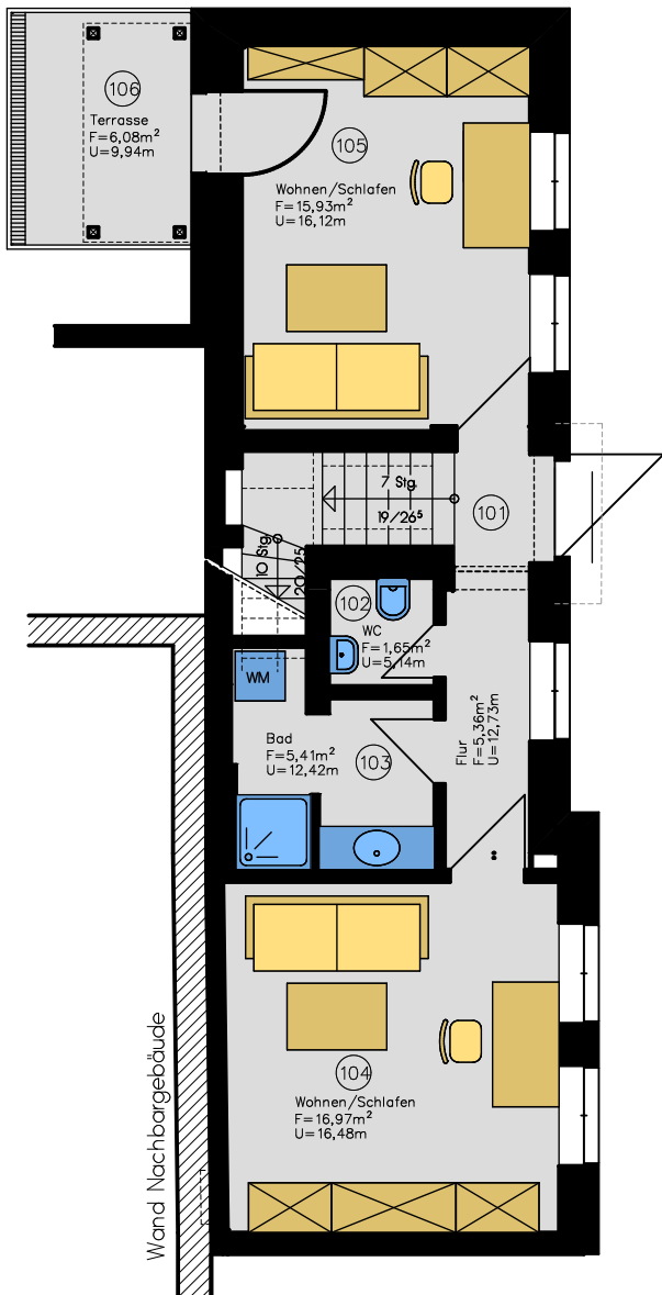
GRUNDRISS EG
